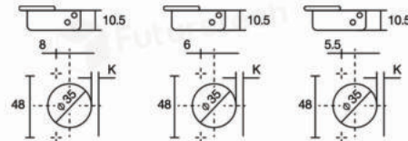
3027090 พลาสติกสำหรับลิ้นคองคา (90 องศา) 0.9x12mm.
